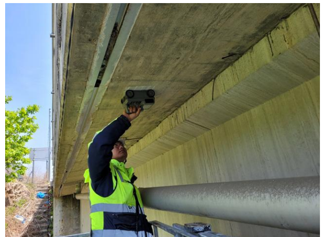
철근탐사
